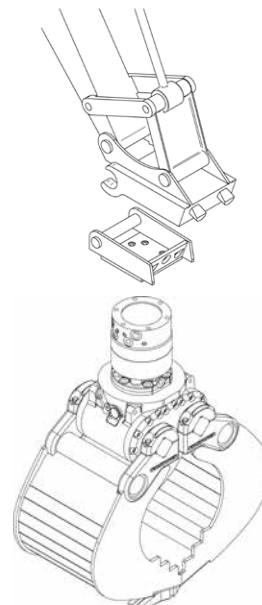
Greifer mit Schraubadapter für Aufnahme an Schnellwechsel-System
